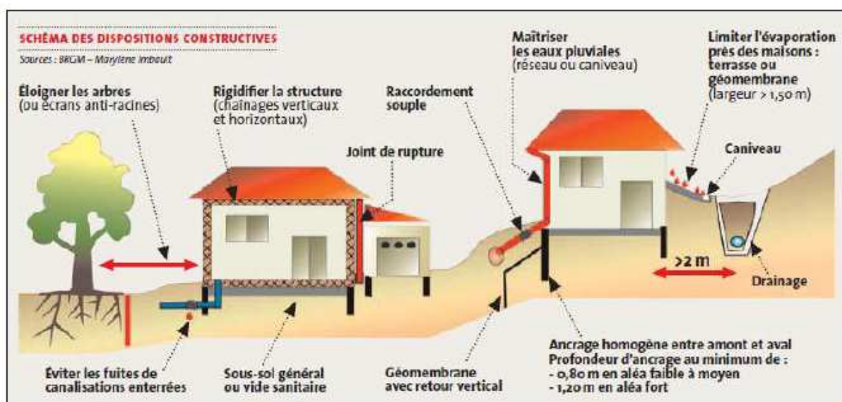
Illustration 6 : Schéma synthétique des dispositions constructives (www.georisques.gouv.fr)
