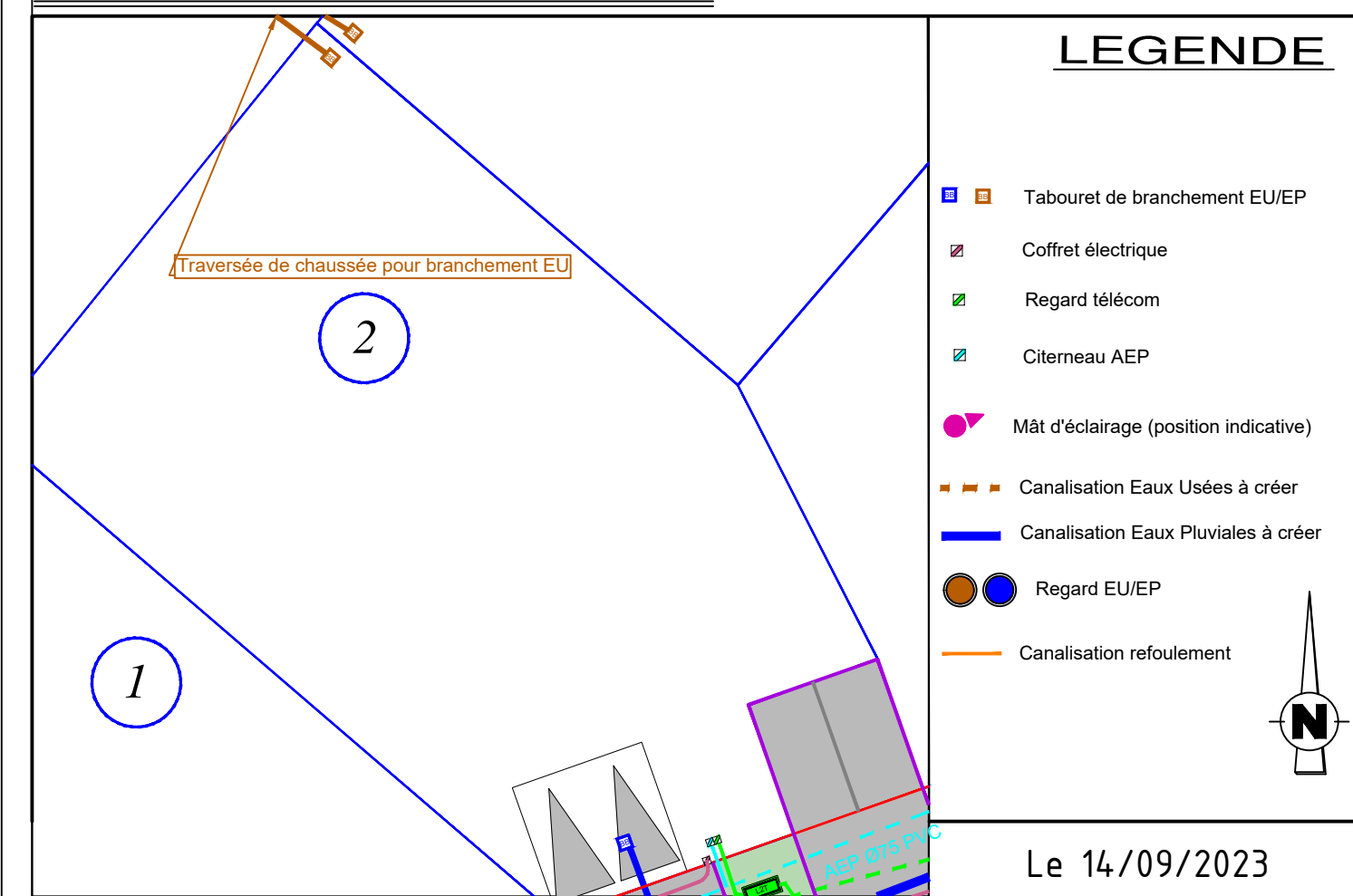
PLAN DES RESEAUX ECHELLE 1 / 250
