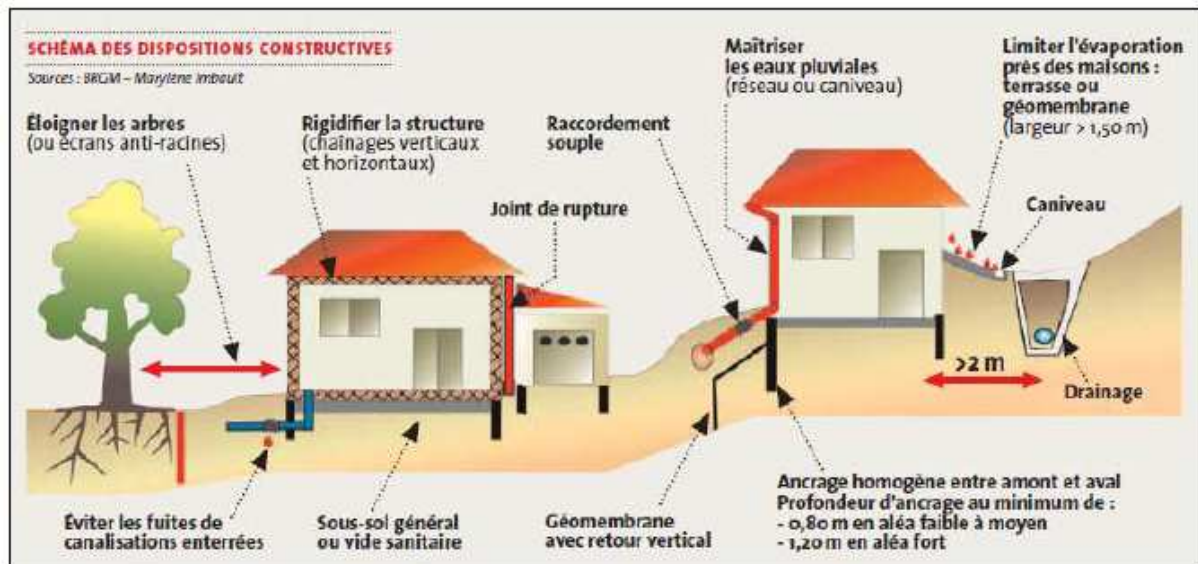
Illustration 4 : Schéma synthétique des dispositions constructives (www.georisques.gouv.fr)
