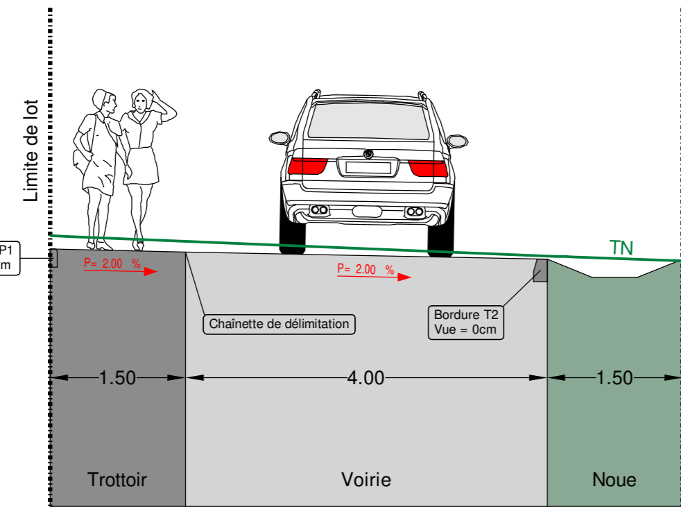
Coupe BB'
