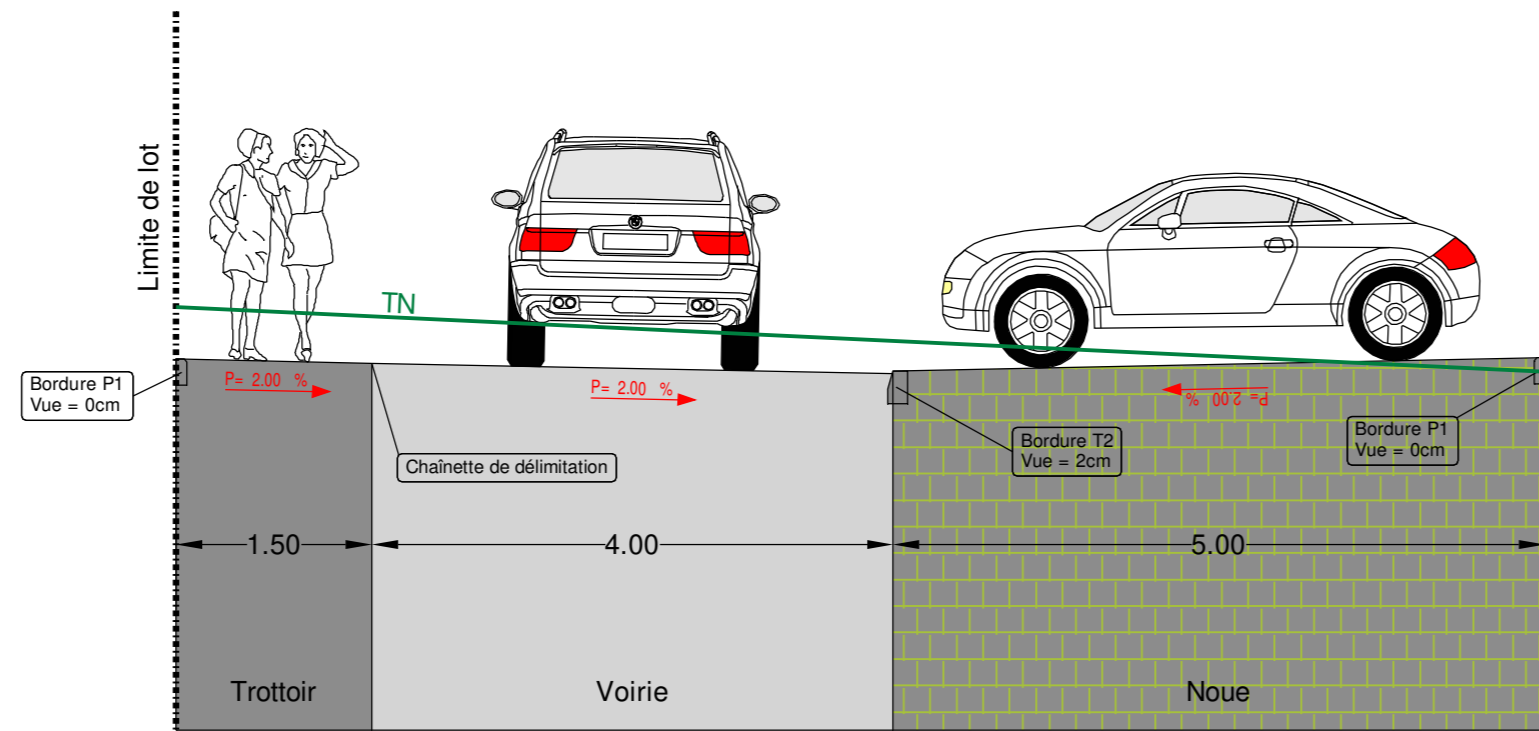
Coupe CC'
