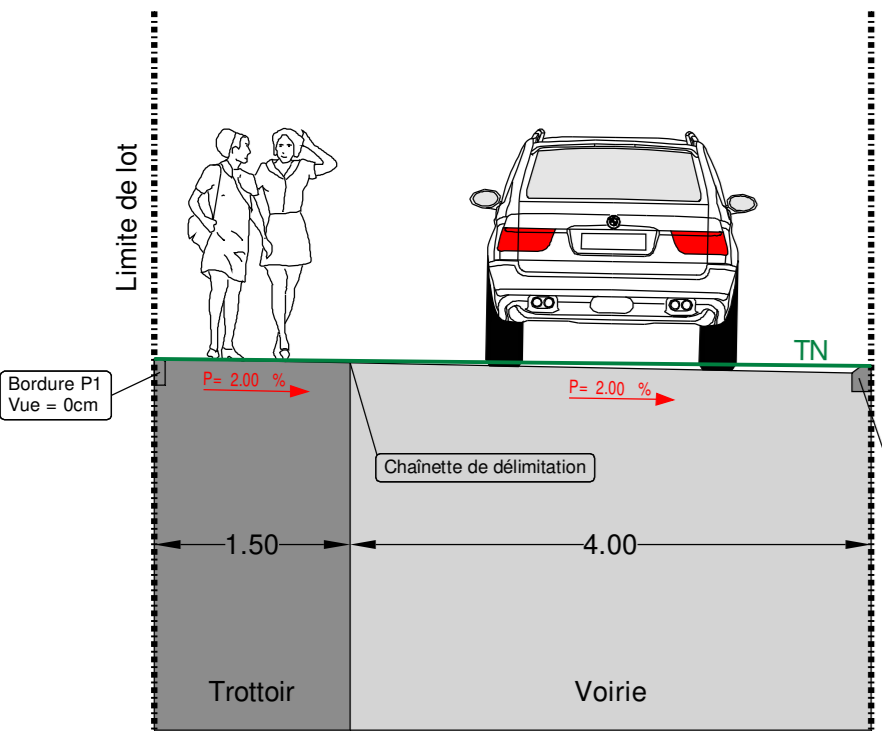
Coupe AA'
