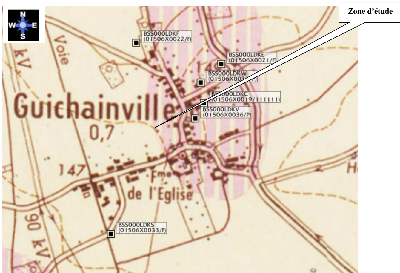
Illustration 3 : Puits et piézomètres à proximité
