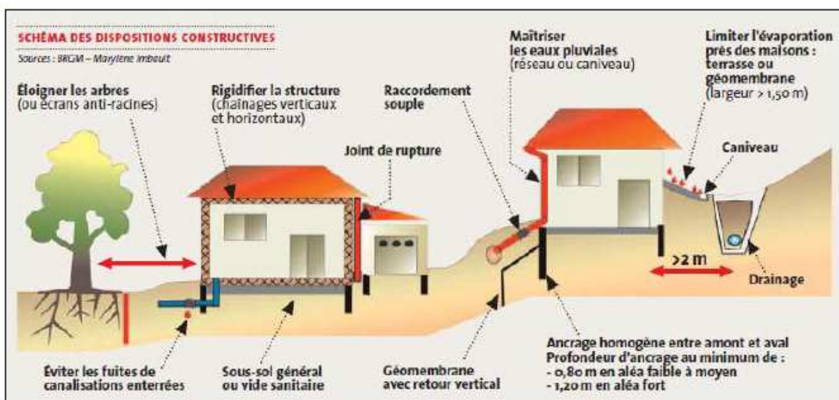
Illustration 7 : Schéma synthétique des dispositions constructives (www.georisques.gouv.fr)
