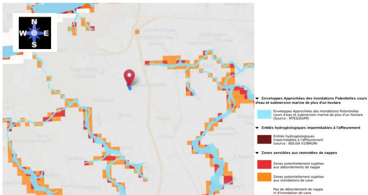
Illustration 5 : Risque de remontées de nappe
