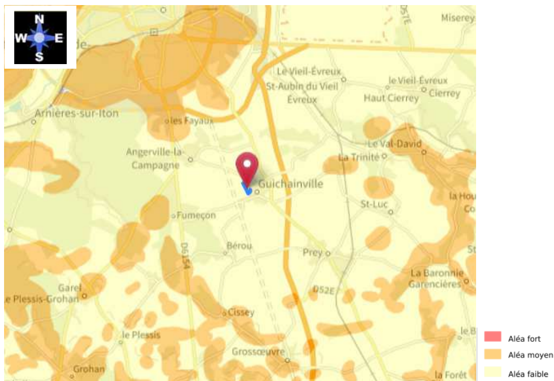
Illustration 4 : Aléa retrait-gonflement des argiles
