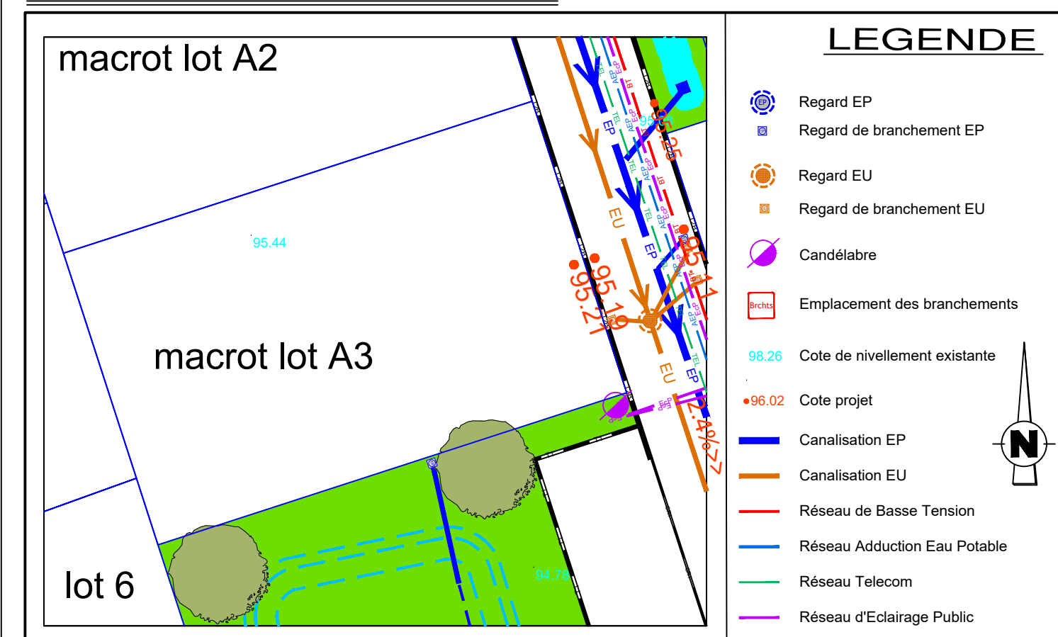
PLAN DES RESEAUX ECHELLE 1 / 500
