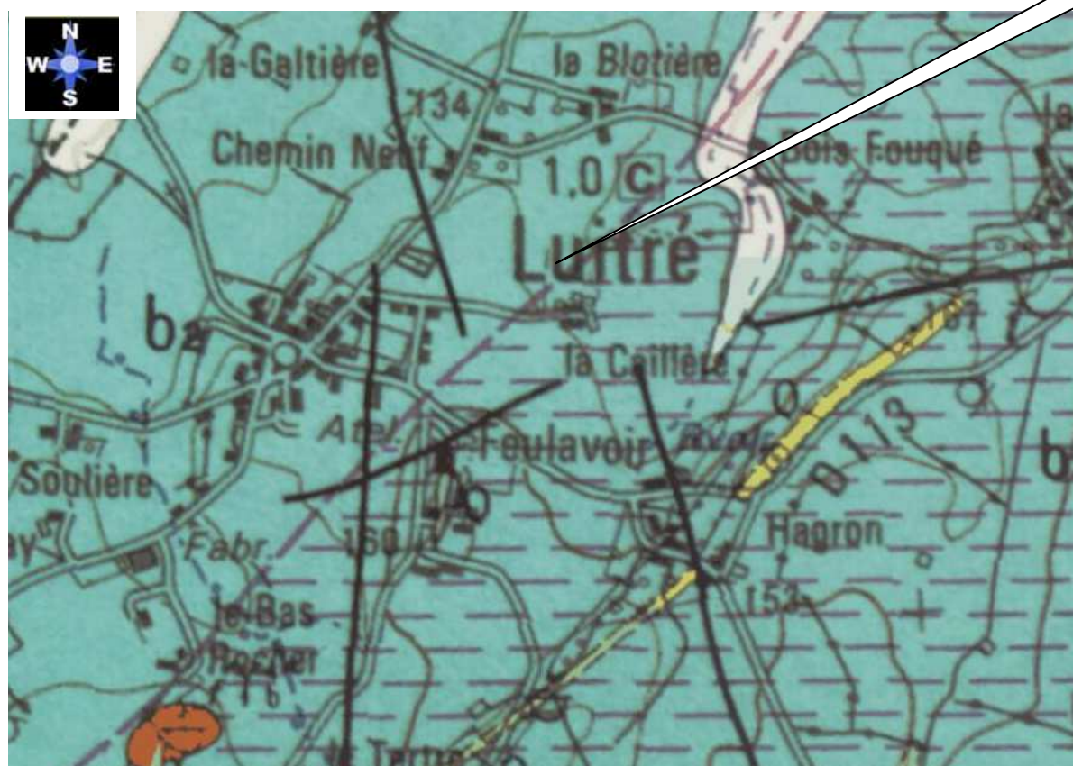
Illustration 2 : Contexte géologique général
