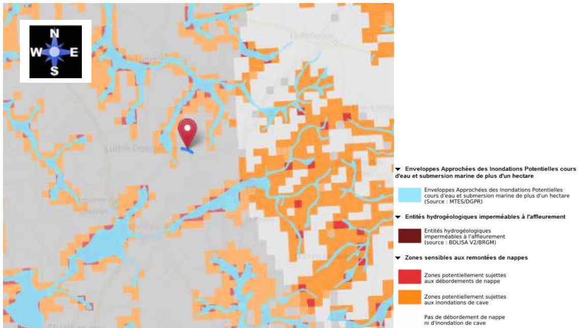
Illustration 4 : Risque de remontées de nappe
