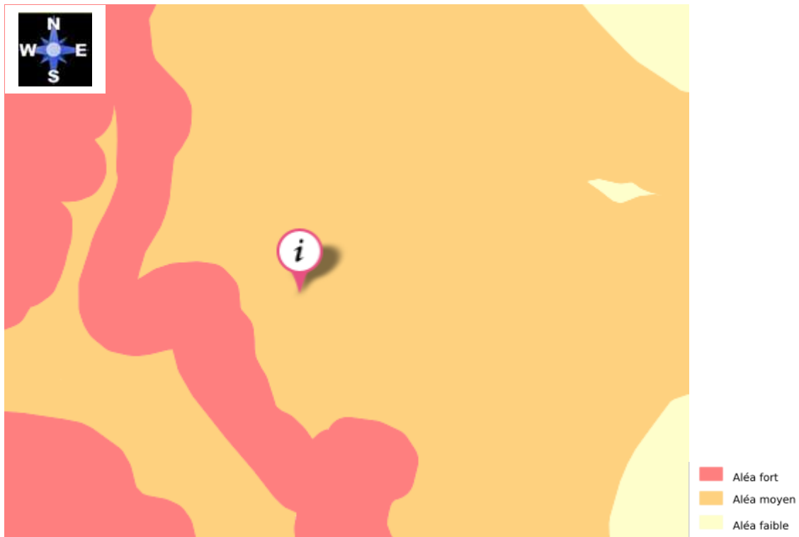
Illustration 3 : Aléa retrait-gonflement des argiles
