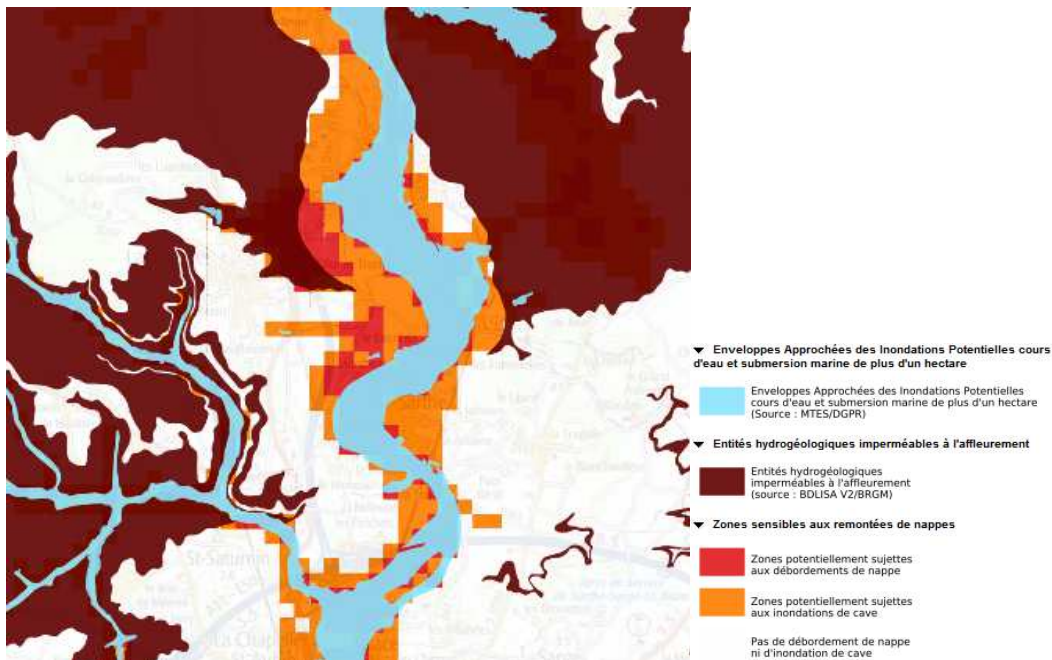
Illustration 4 : Risque de remontées de nappe
